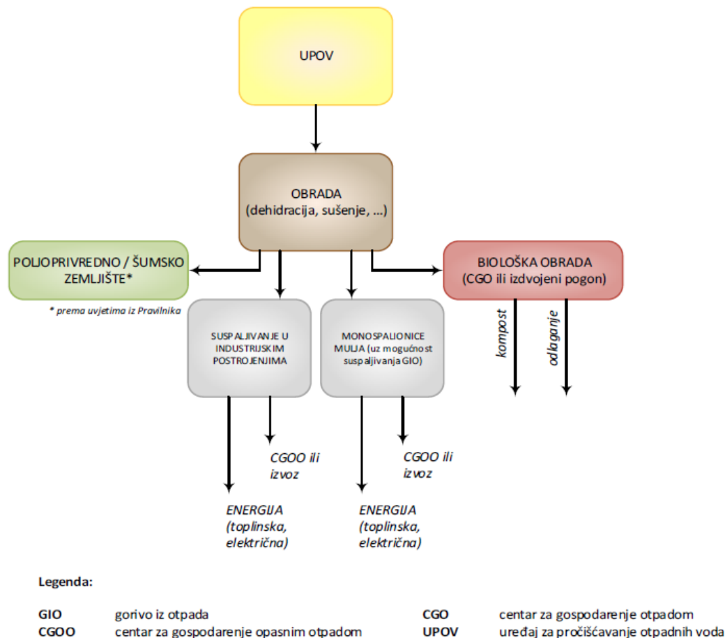
Shema 3. Gospodarenja otpadnim muljem iz uređaja za obradu otpadnih voda
